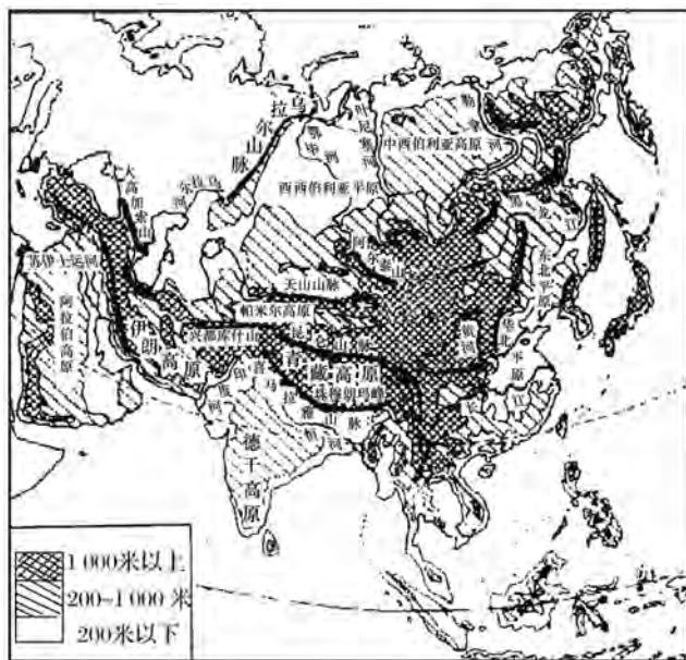
亚洲地形图
