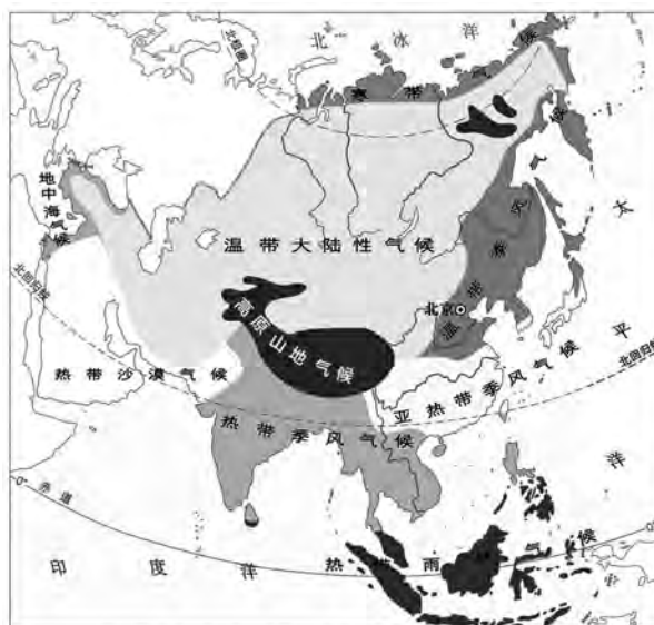
亚洲气候图
