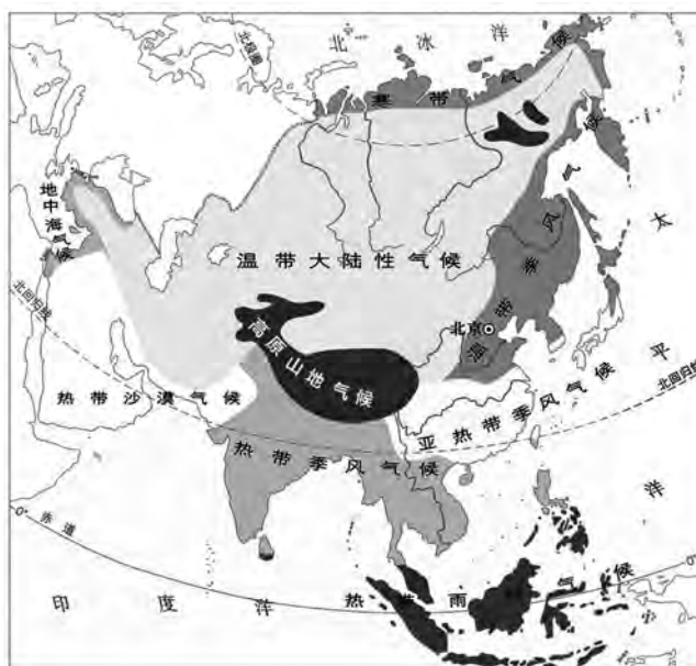
亚洲气候图
