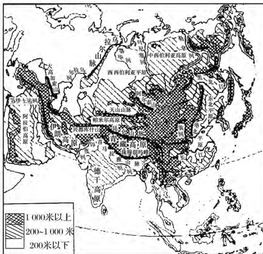
亚洲地形图
